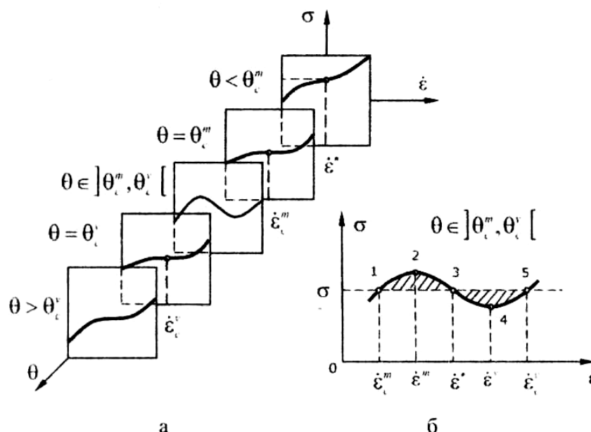
Рисунок 1 – Схематическое представление экспериментальных зависимостей «напряжение-скорость деформации» алюминиевых сплавов в различных температурных диапазонах (а); к условиям перехода алюминиевых сплавов в сверхпластическое состояние (б)
