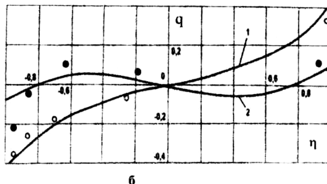
Рисунок 2 – Сопоставление теоретических (сплошные линии) и экспериментальных (○, ●) данных при растяжении и сжатии образцов: а) сплав: АМг5 при: 1 (○) – \theta = 713 \text{ K} ; m_0 = 0,3333 ; \beta = 0,1727 ; 2 (●) – \theta = 753 \text{ K} ; m_0 = 0,3333 ; \beta = -0,0335 ; б) сплав: АК4 при: 1 (○) – \theta = 723 \text{ K} ; m_0 = 0,2428 ; \beta = 0,1733 ; 2 (●) – \theta = 783 \text{ K} ; m_0 = 0,2428 ; \beta = -0,1679
