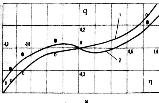
Рисунок 2 – Сопоставление теоретических (сплошные линии) и экспериментальных (○, ●) данных при растяжении и сжатии образцов: а) сплав: АМг5 при: 1 (○) – \theta = 713 \text{ K} ; m_0 = 0,3333 ; \beta = 0,1727 ; 2 (●) – \theta = 753 \text{ K} ; m_0 = 0,3333 ; \beta = -0,0335 ; б) сплав: АК4 при: 1 (○) – \theta = 723 \text{ K} ; m_0 = 0,2428 ; \beta = 0,1733 ; 2 (●) – \theta = 783 \text{ K} ; m_0 = 0,2428 ; \beta = -0,1679
