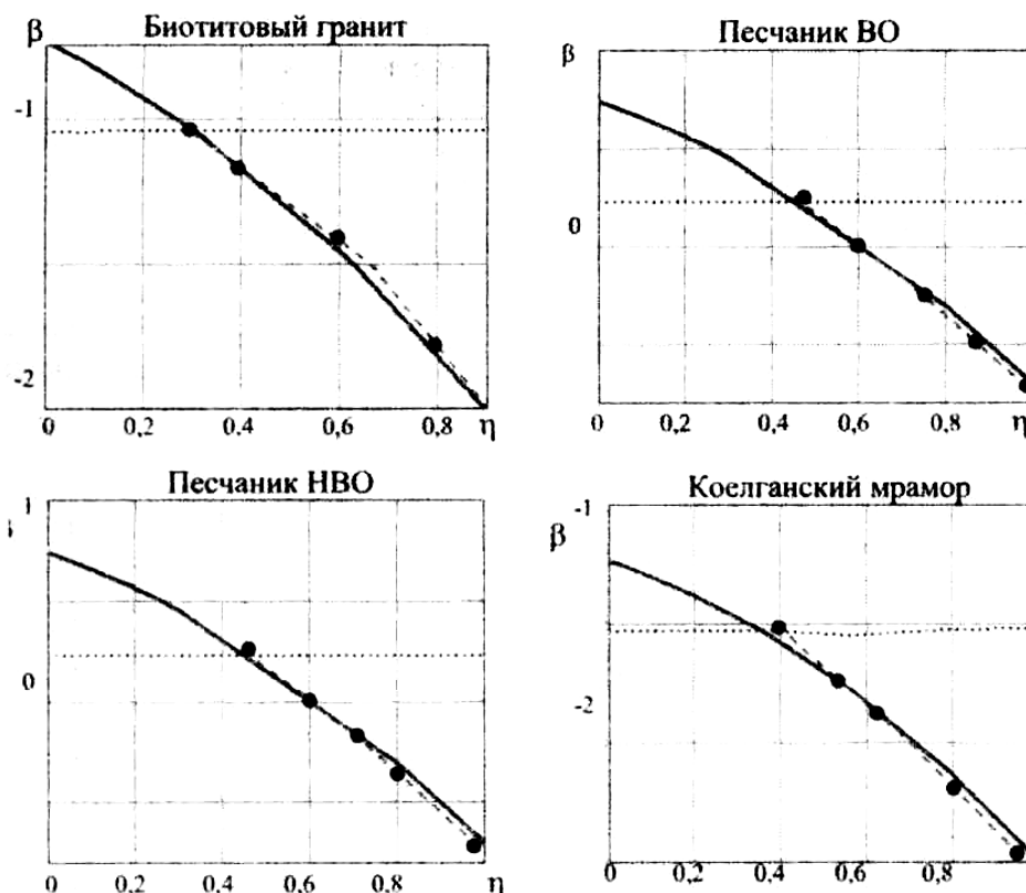
Рисунок 4 – Сопоставление экспериментальных и теоретических данных
