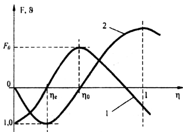
Рисунок 3 – График закономерностей деформирования горных пород
